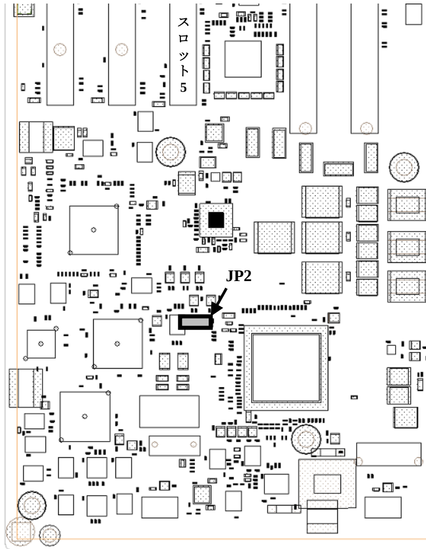
図 6 - 1 7 JP2実装位置
