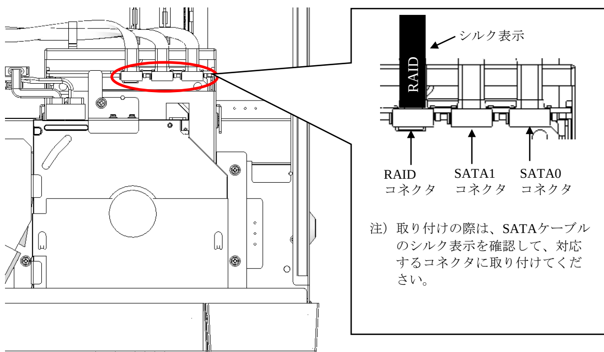
図6-4 SATAケーブルの取り外し
