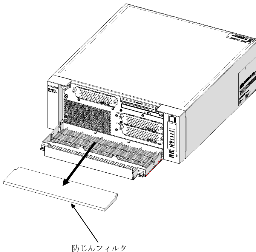
図6－15 防じんフィルタの交換
