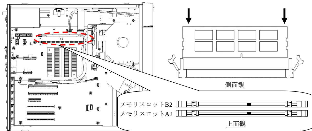
図6-5 メインメモリの取り付け
