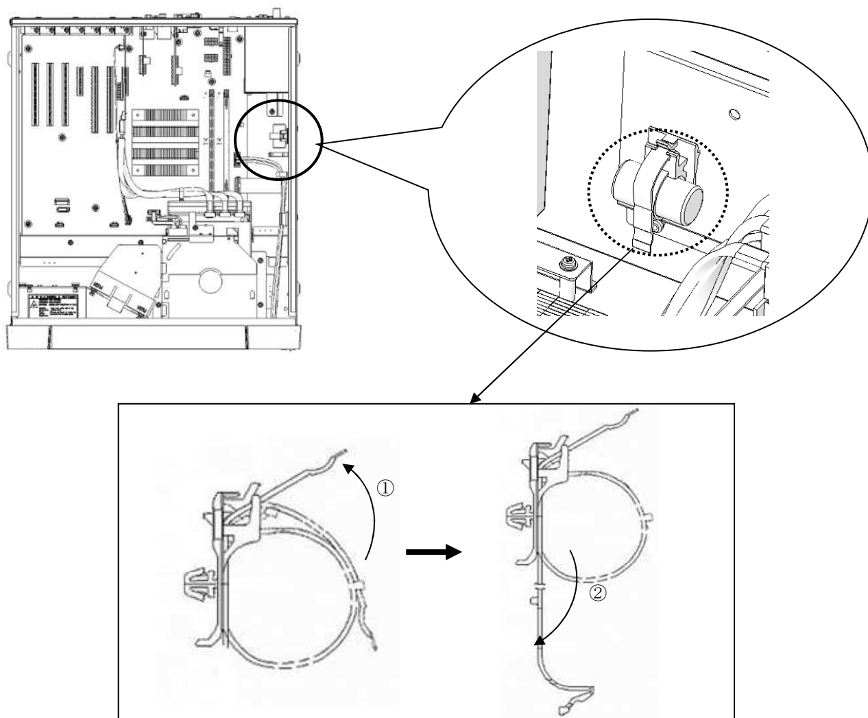
図6-16 リチウム電池の取り外し
