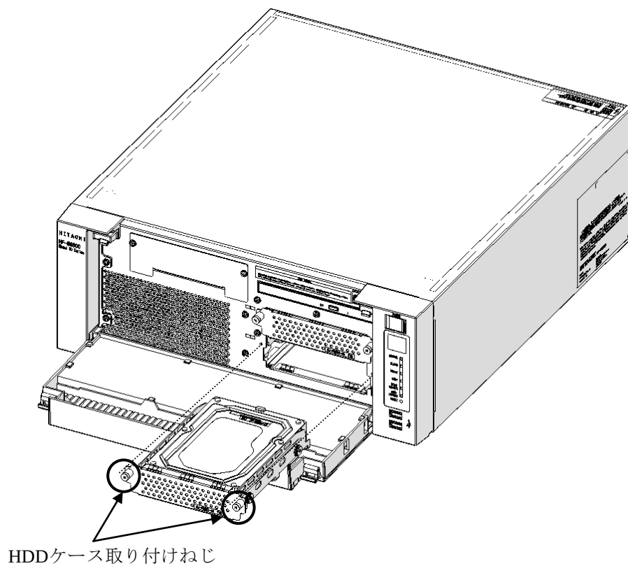
図6-7 HDDの取り外し
