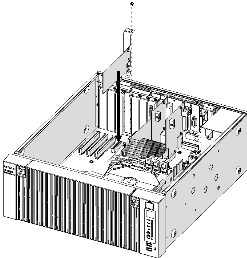
図 6-3 拡張ボードの取り付け
