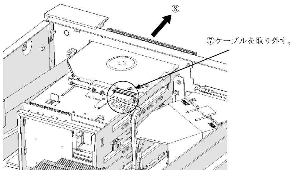
図6-11 DVDドライブの取り外し
