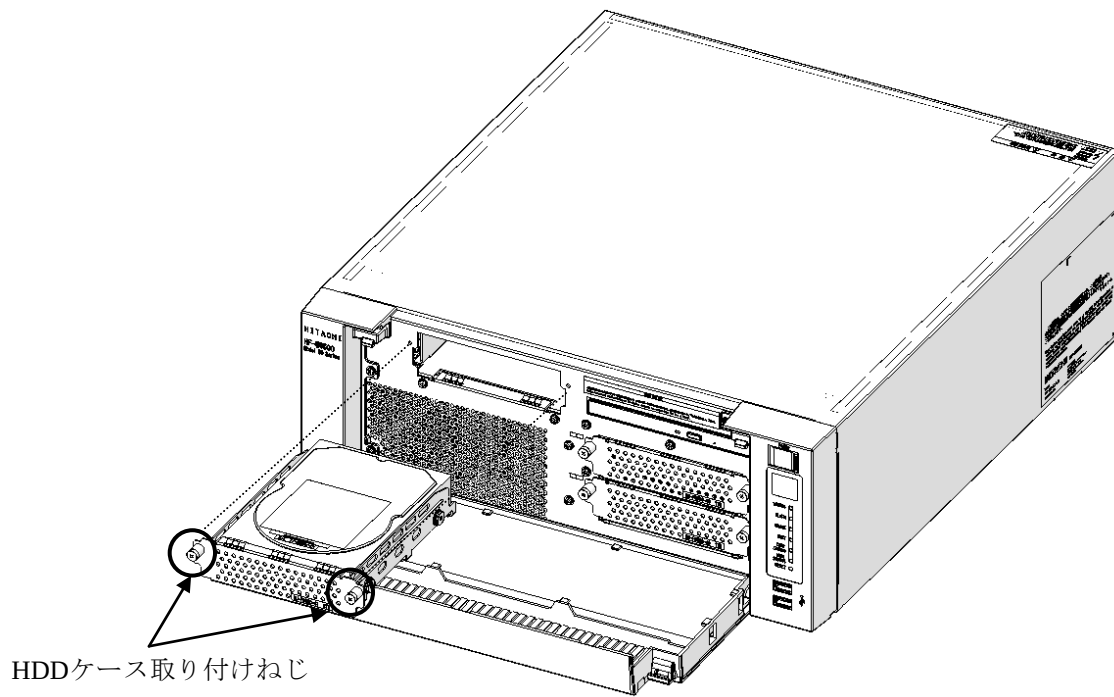
図6-8 HDDドライブベイ3 HDDの取り外し
