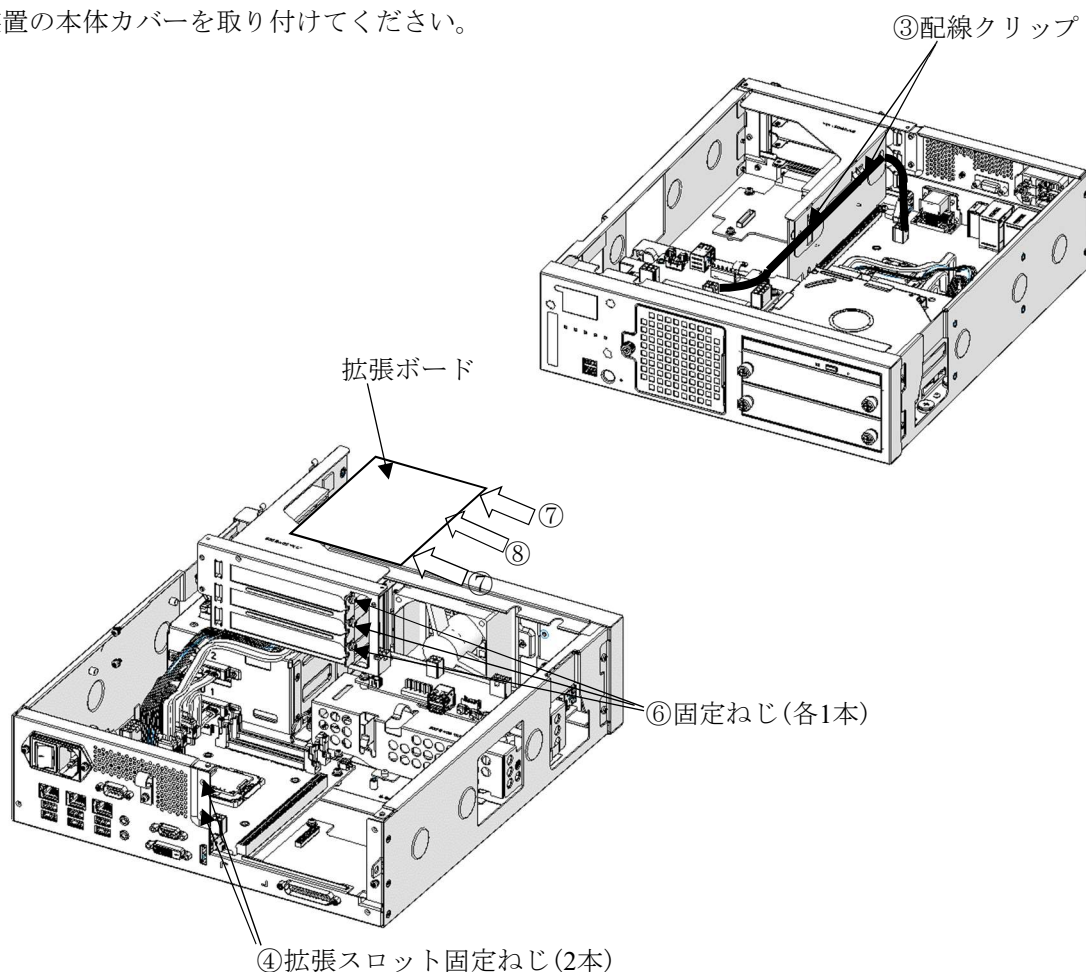
図6-4 拡張ボードの取り付け
