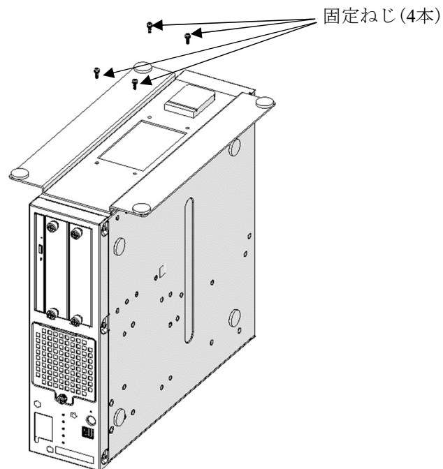
図6－11 縦置きスタンドの取り付け
