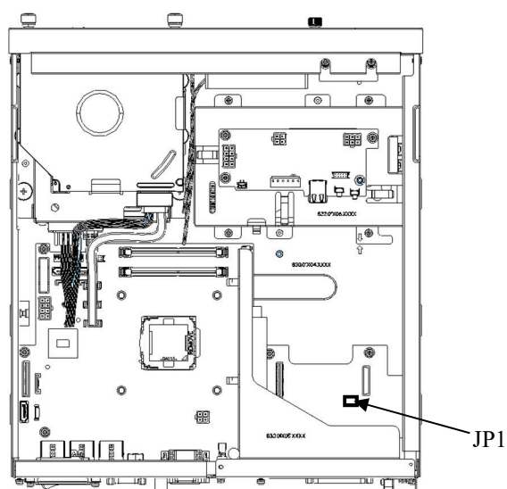
図6-13 JPソケットの取り外し
