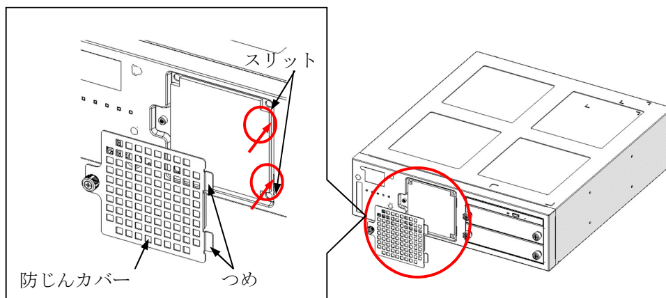
図6－10 防じんフィルタの取り付け
