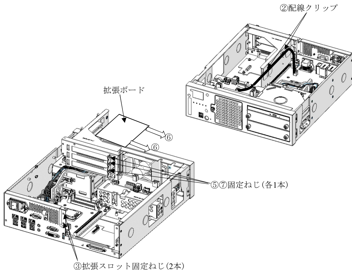
図6-5 拡張ボードの取り外し
