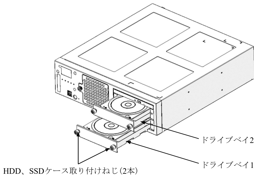
図6-7 HDD、SSDの取り外し
