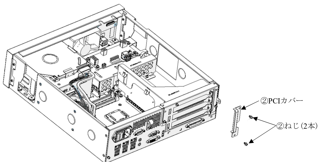
図6-3 PCIカバーの取り外し
