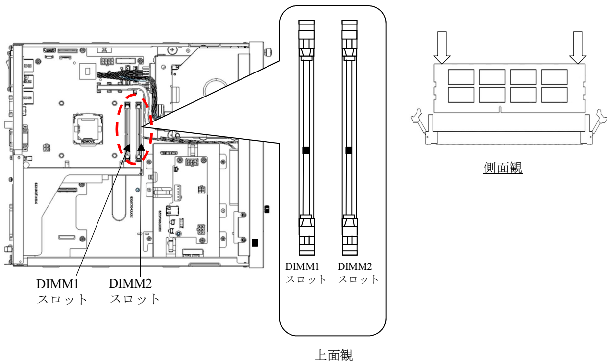
図6-6 メインメモリの取り付け
