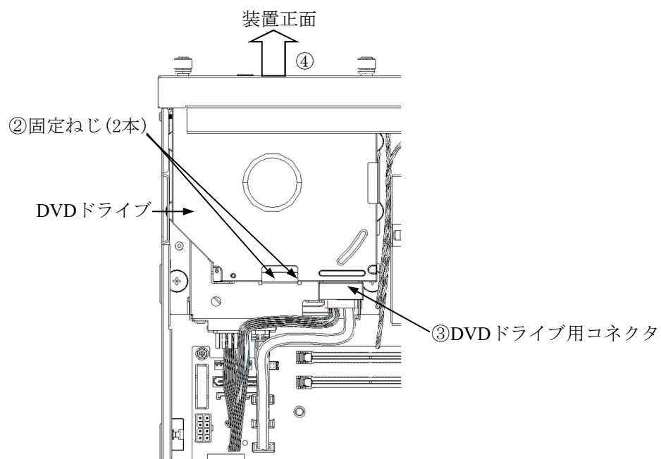
図6－8 DVDドライブの取り外し
