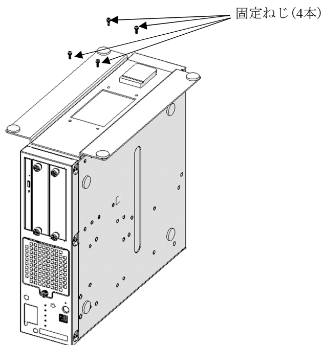
図6-11 縦置きスタンドの取り付け
