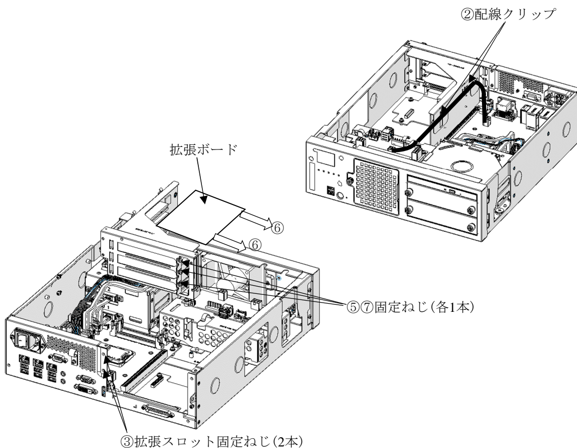
図6-5 拡張ボードの取り外し
