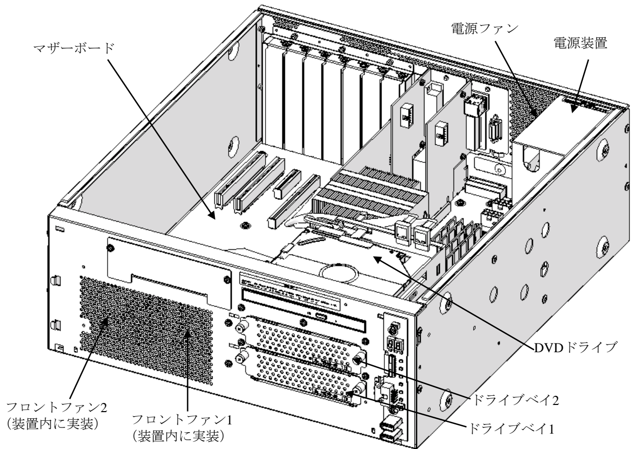
図1-3 装置内実装構成
