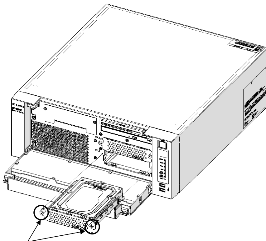
図6-7 HDD/SSDの取り外し
