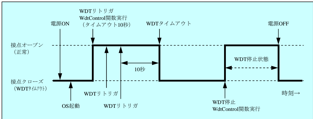
図6-1 WDTTO接点の動作
