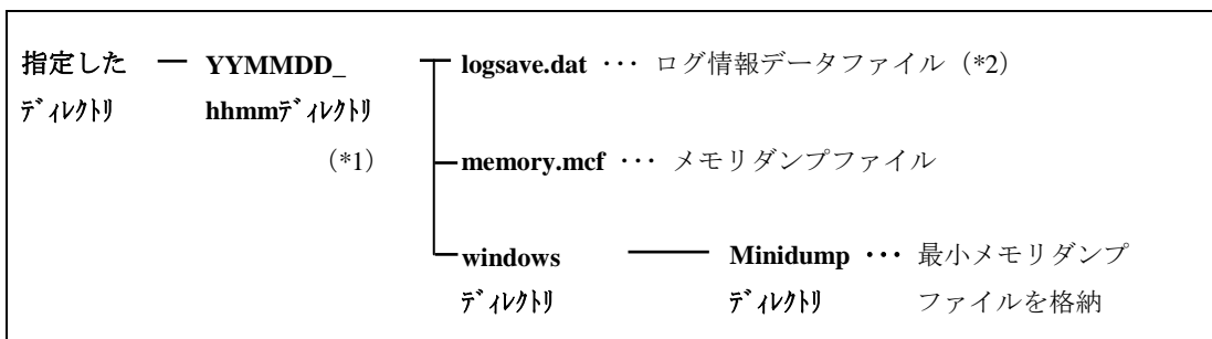
図7-1 収集結果のフォルダ構成
